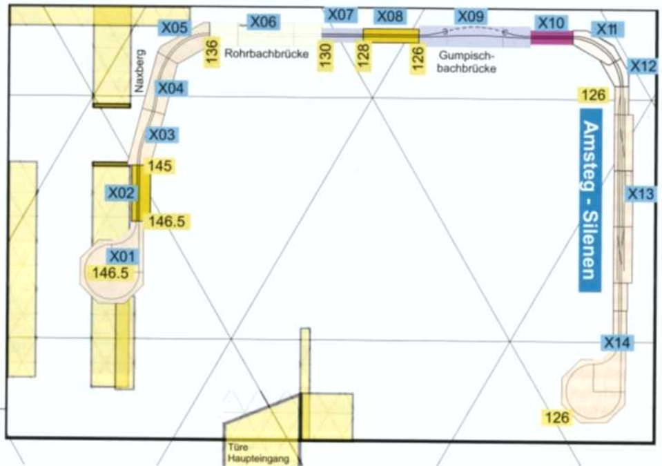
Anlagenplan-Grundriss des Vereinslokals mit 23-teiliger Modulanlage.
